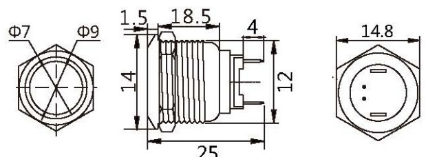
GQ12F-10EJN 电源标志带灯自锁款
